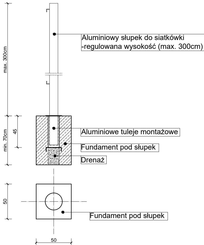
SŁUPEK DO SIATKI SIATKÓWKI Ruchomy (Detal 1.2)
