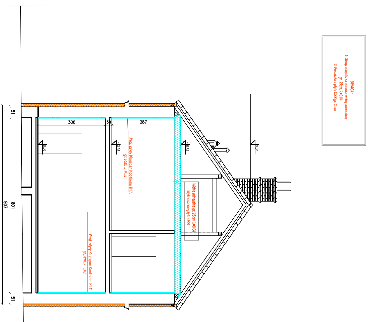
PRZEKRÓJ C – C
