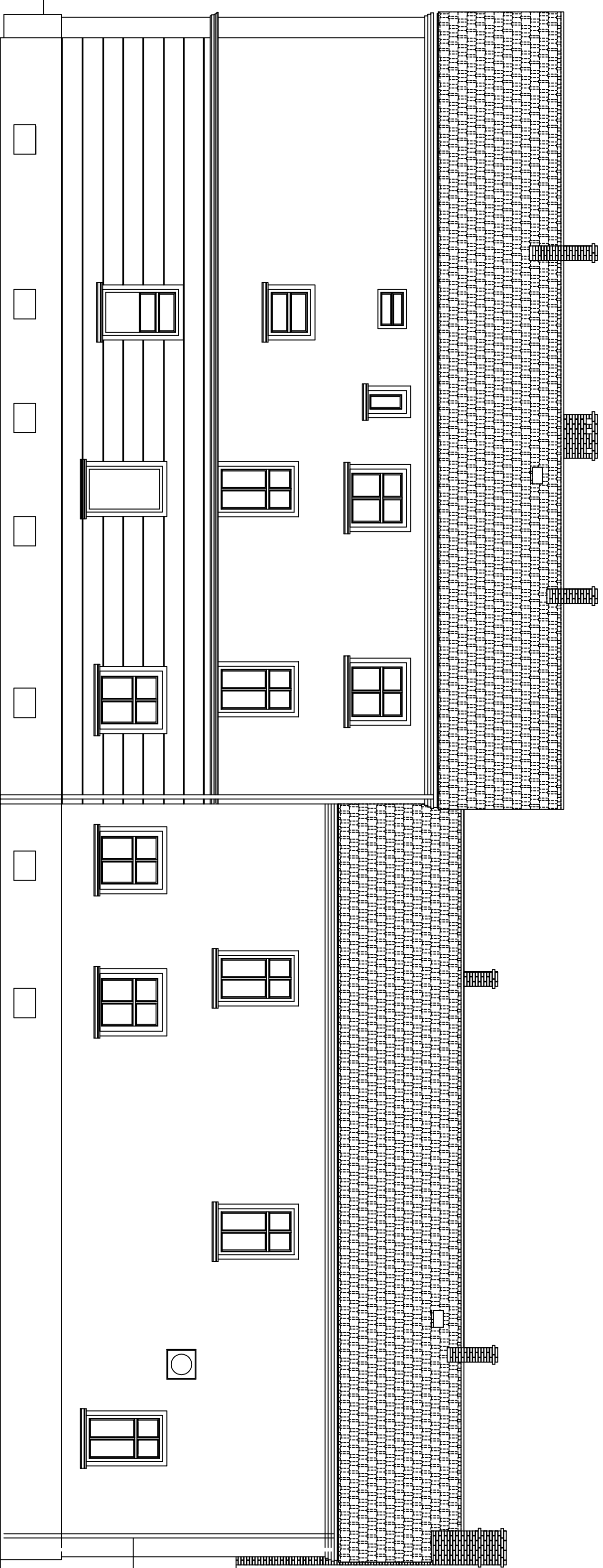
ELEWACJA PÓLNOCCNO – ZACHODNIA
